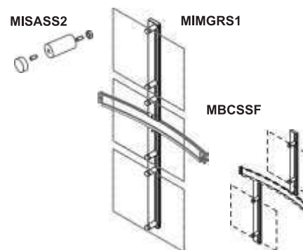
Панели на дистанционных держателях.
